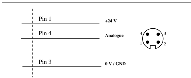
Wiring/Anschlüsse/Raccordement électrique
